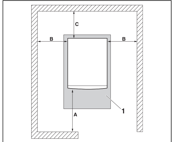
Fig. 7 Distanțe față de perete în încăperea centralei termice
