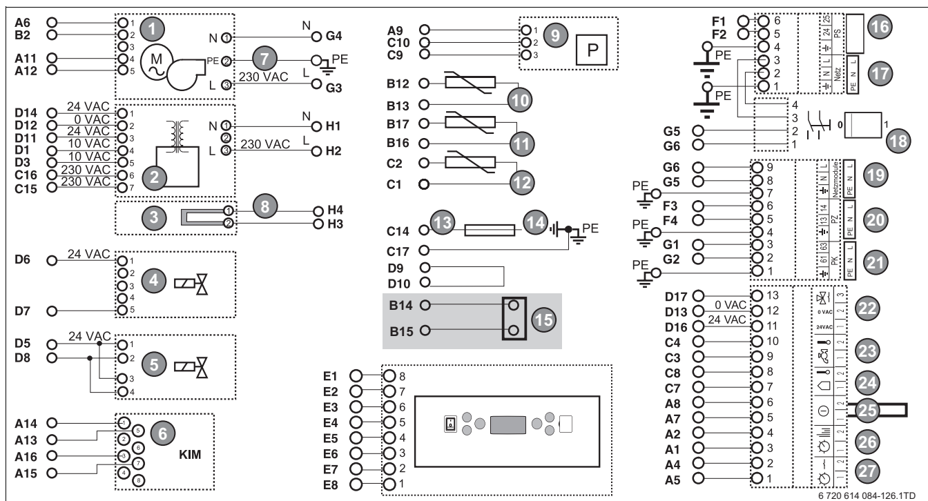
Fig. 5 Schemă de conexiuni
