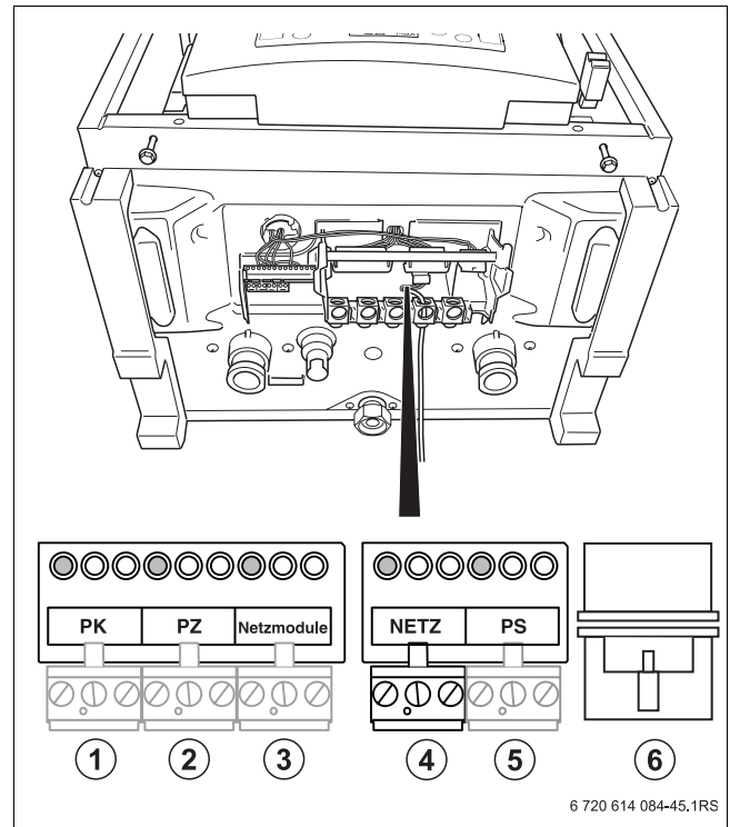
Fig. 22 Cutie de racordare
