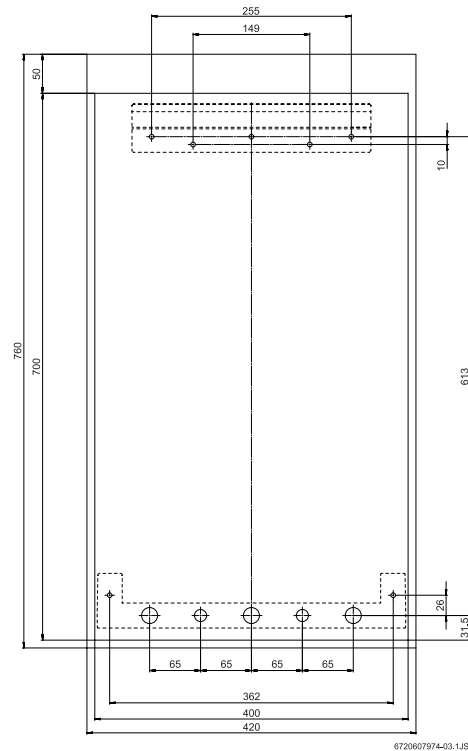
Fig. 8 Ansamblu de montaj pe perete
