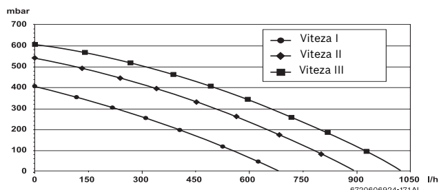
Fig. 6 Caracteristica pompei
